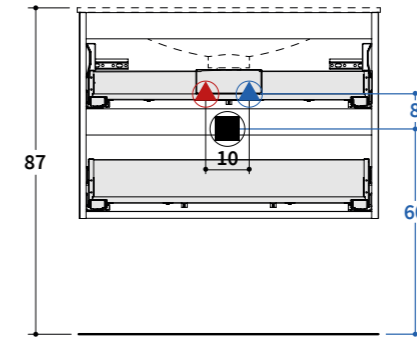
VISTA FRONTALE Frontal view / Vue frontale / Frontalansicht / Vooraanzicht
