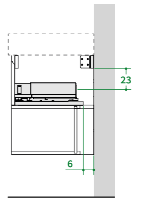
VISTA IN SEZIONE Lateral view / Vue latérale / Seitenansicht / Zijaanzicht
