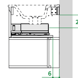
VISTA IN SEZIONE Lateral view / Vue latérale / Seitenansicht / Zijaanzicht
